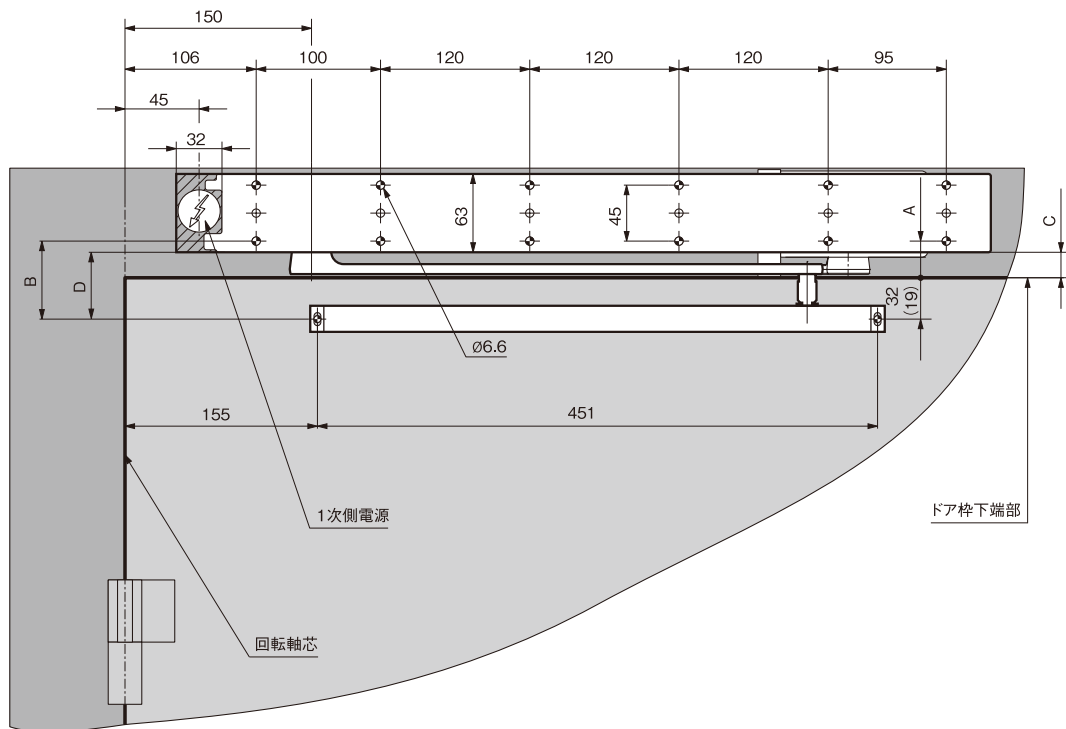
設置箇所断面
